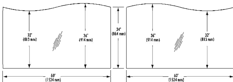
747W-060360L
